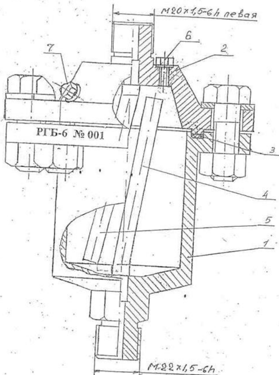
1. Корпус. 2. Крышка. 3. Прокладка. 4. Канал подачи рабочей жидкости. 5. Канал подачи разделительной жидкости. 6, 7. Винты дренажные.
